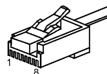
Rys. 8-9 Wtyk RJ45
