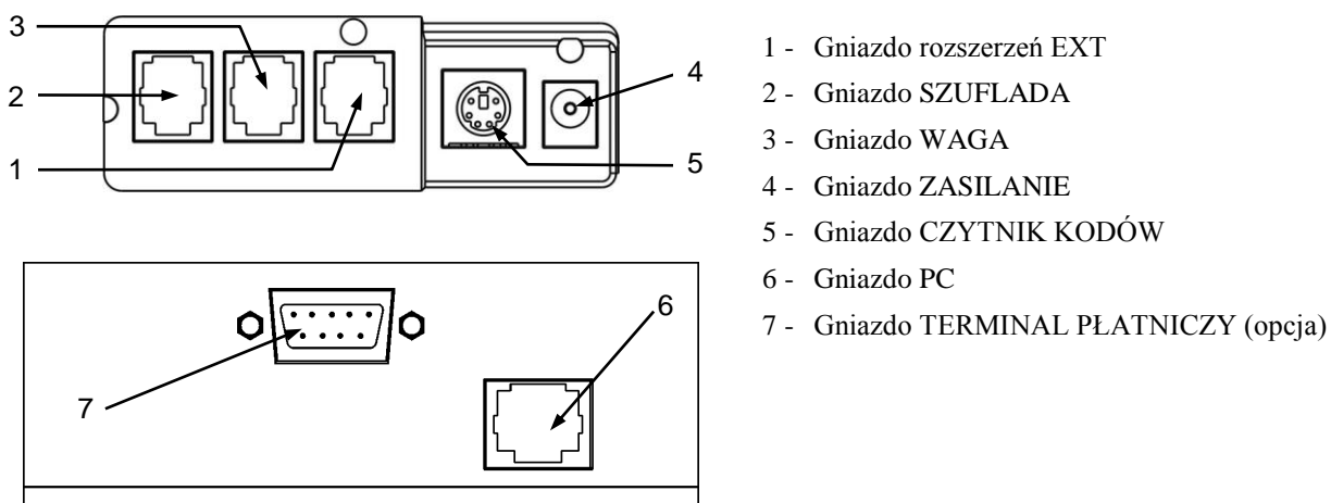
Rys. 1-2 Widok na złącza interfejsów (od spodu kasy)
