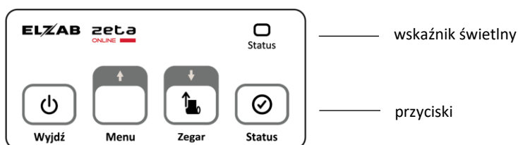
Klawiatura drukarki
