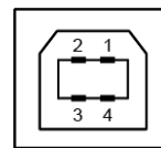
Złącze USB-B
